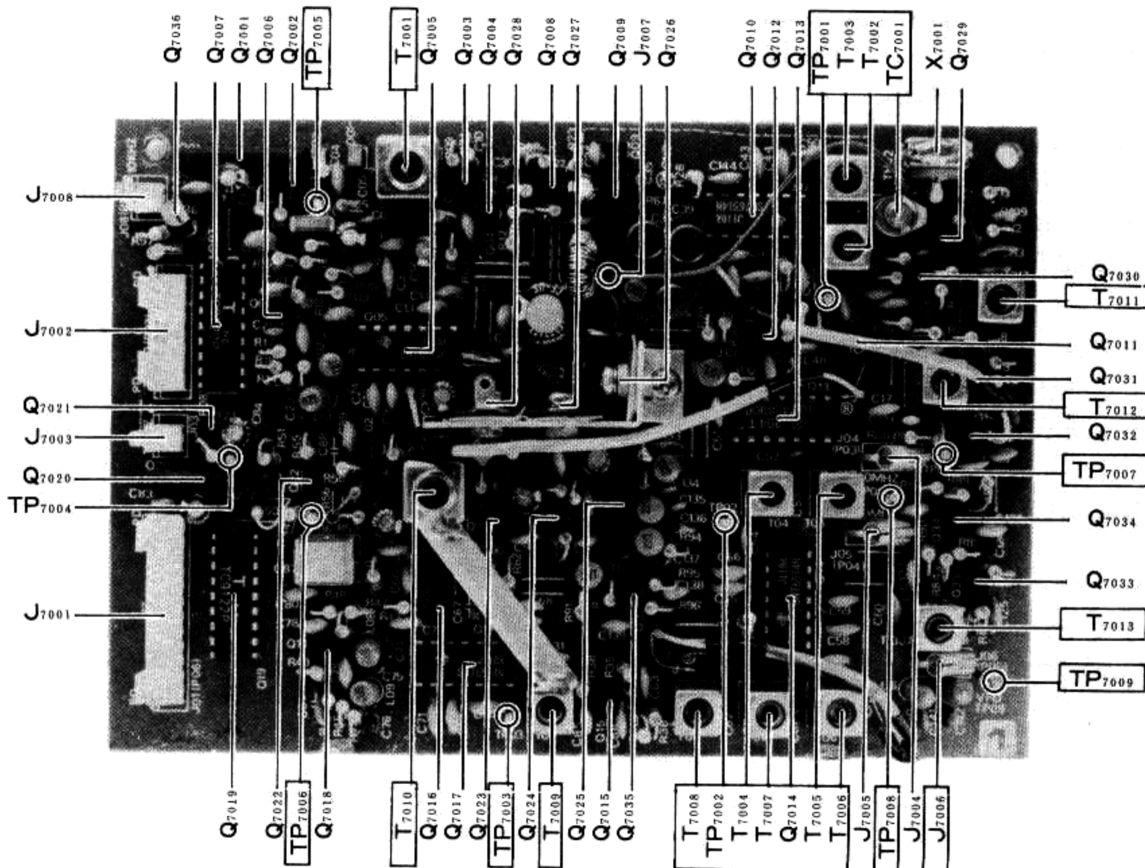
VFO UNIT
