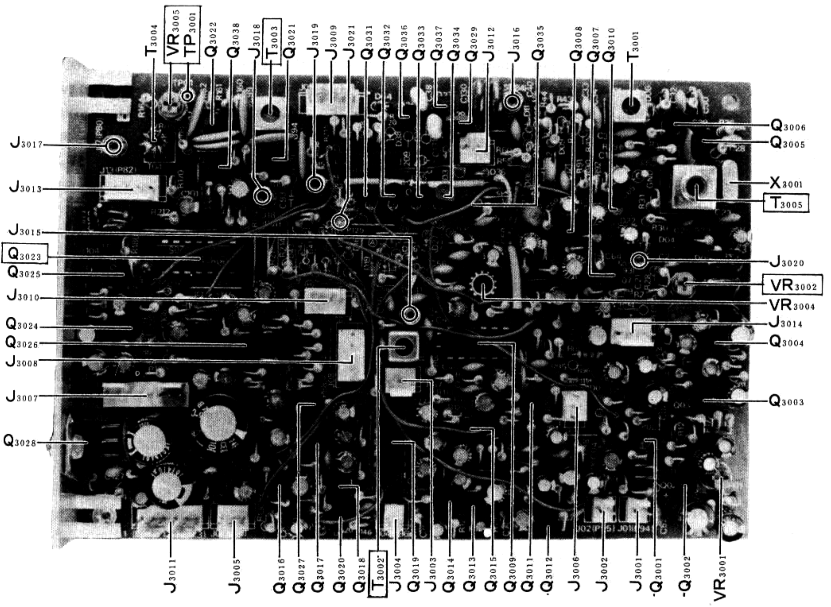
AF UNIT
